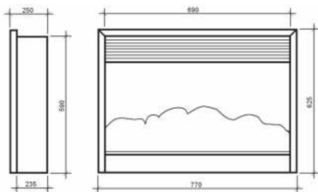
Рис. 1. Внешние размеры указаны для Jupiter Black, Brass.
